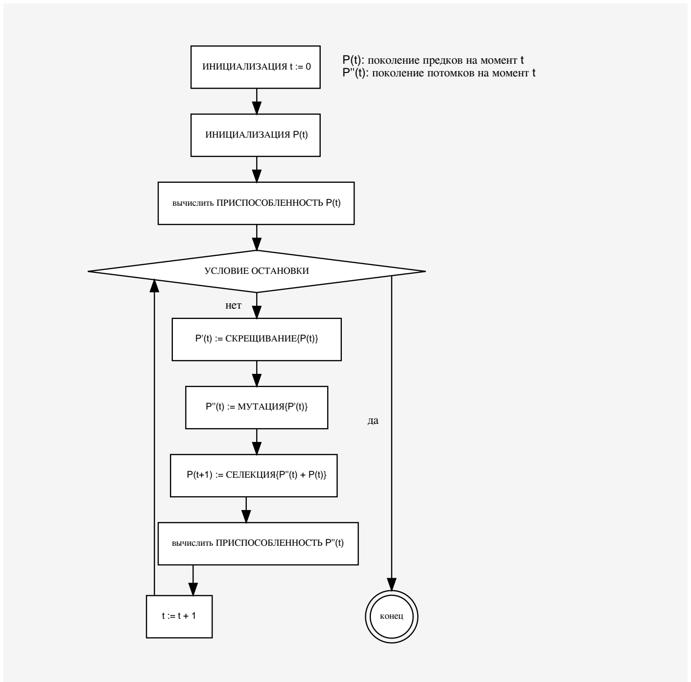
Рисунок 60.1. Структура генетического алгоритма
