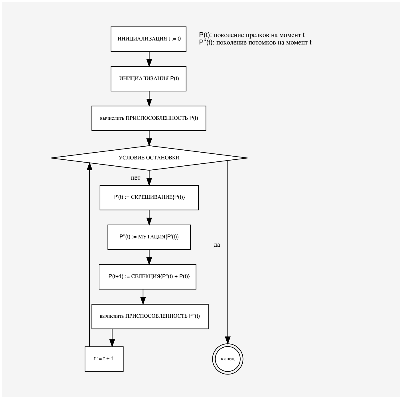
Рисунок 59.1. Структура генетического алгоритма
